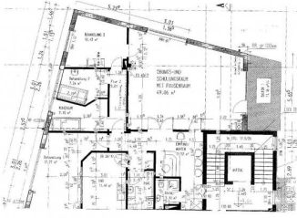
Grundriss
